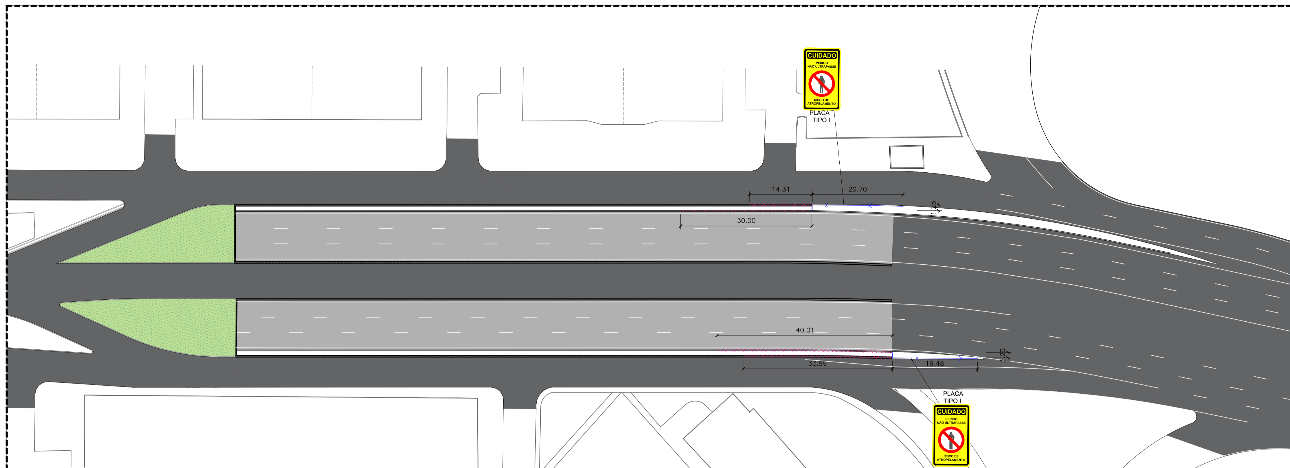
EMBOQUE – SENTIDO EPTG LOCALIZAÇÃO PLACAS DE ADVERTÊNCIA ESC. 1:500
