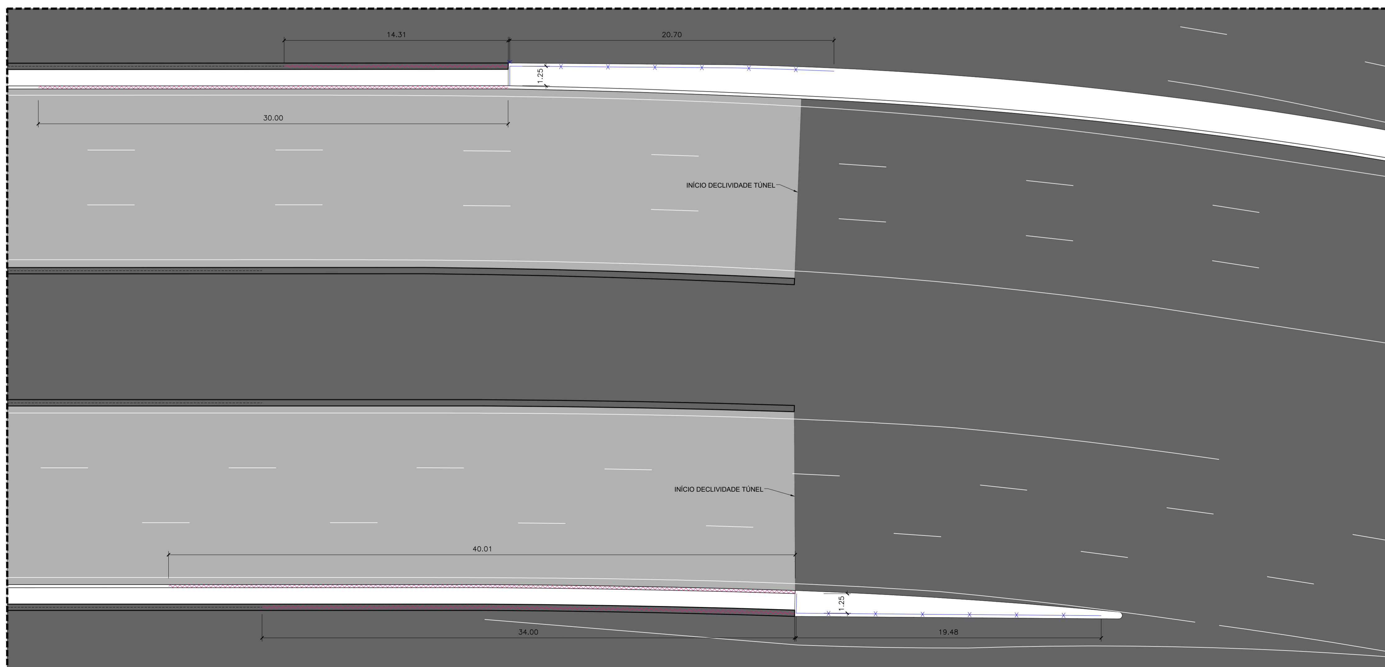
EMBOQUE – SENTIDO EPTG ESC. 1:150
